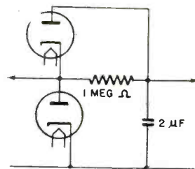
Modified rectifier circuit
